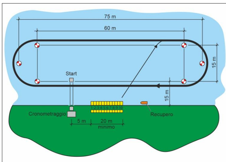
Disegno 6 – Eco (le misure da considerarsi minime)
