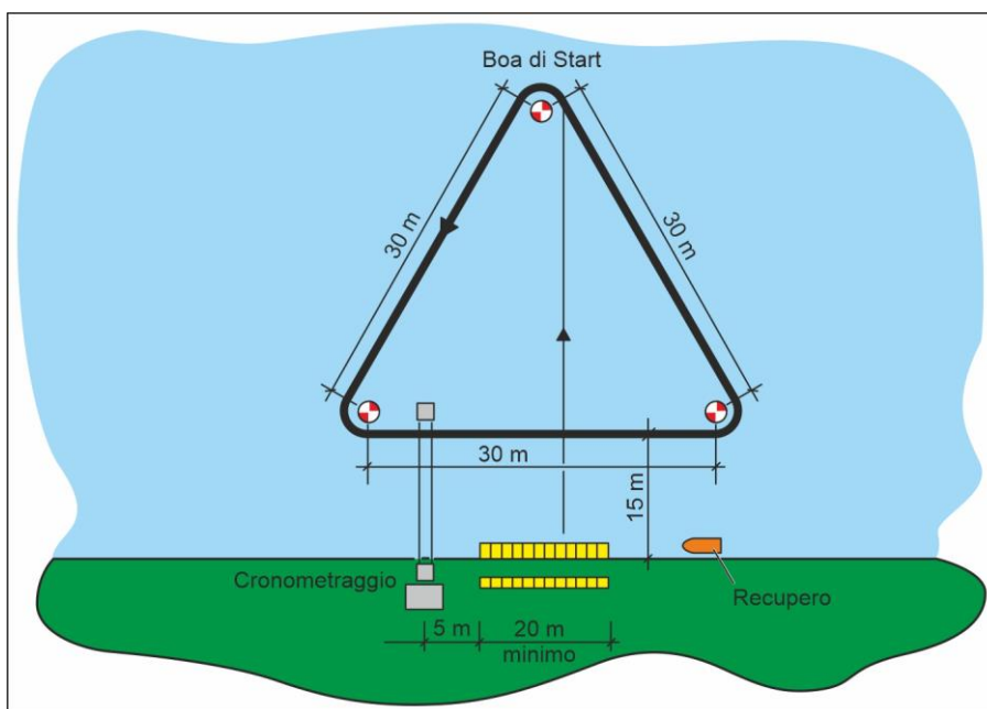
Disegno 6 – Eco (le misure da considerarsi minime)
